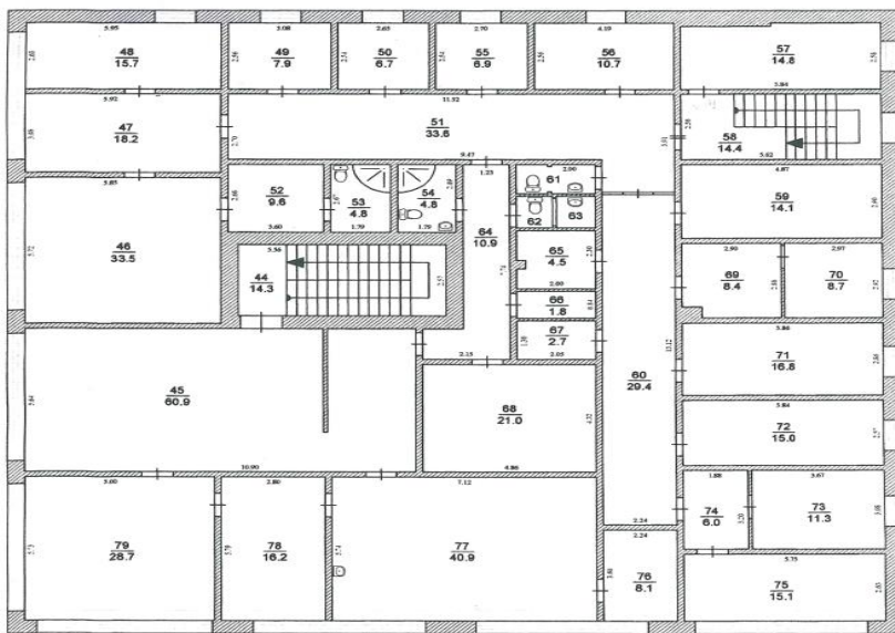
Второй этаж
